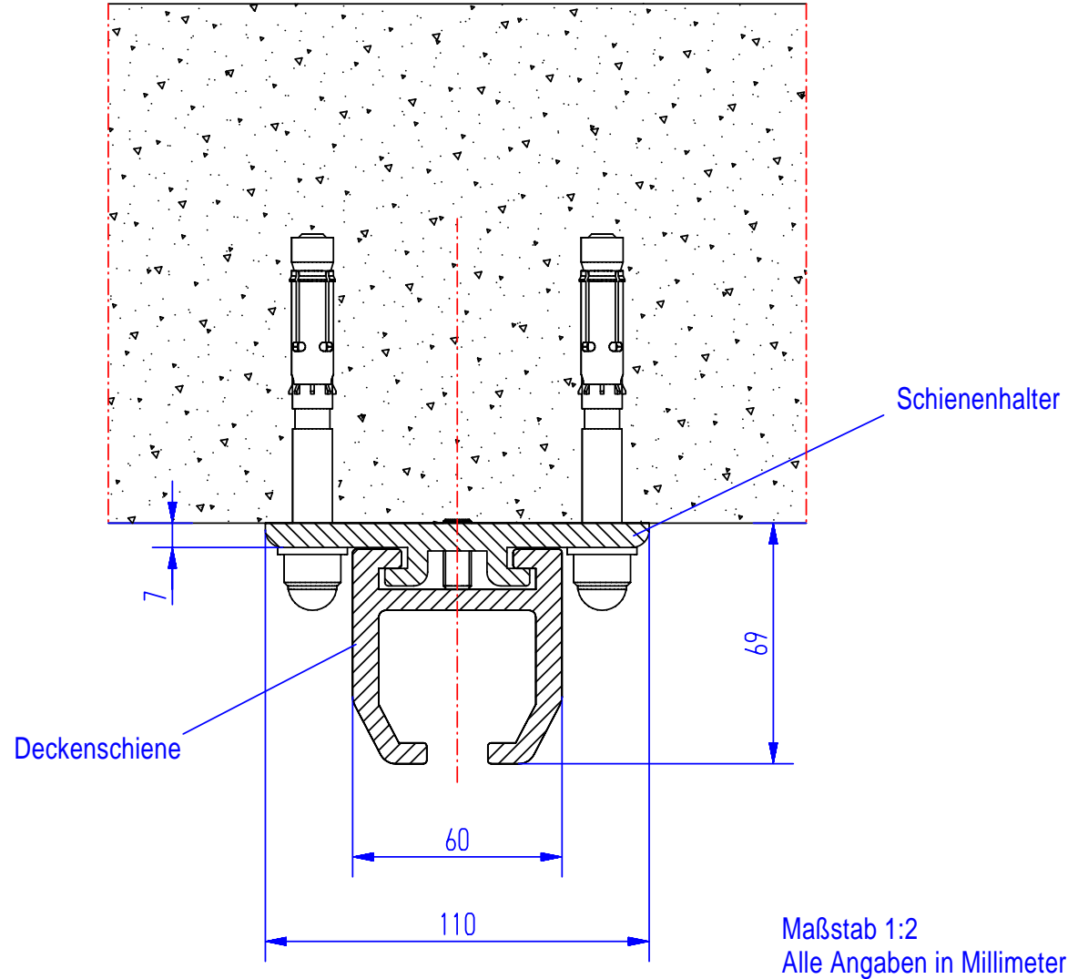
Deckenschiene mit Schienenhalter
