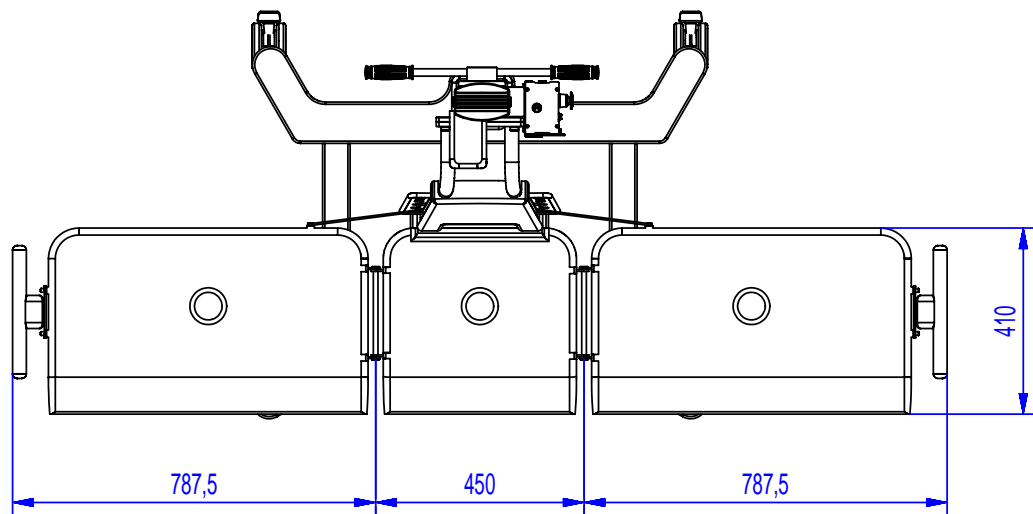
Maßzeichnung für Mona Badeliege mit Raumspar-Handgriff
